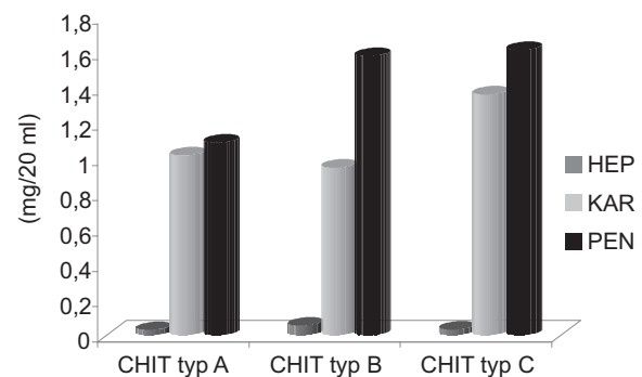
Graf 1. Uvoľnené množstvo liečiv po 180. min z hydrogélov na báze troch typov CHIT
