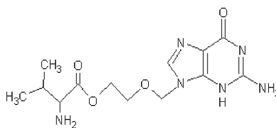
Obr. 2. Struktura valacikloviru
