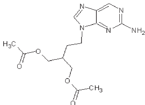
Obr. 3. Struktura famcicloviru
