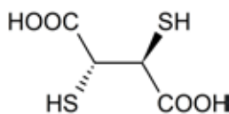
Obr. 3. Štruktúra DMSA (kyseliny dimerkaptojantárovej)
