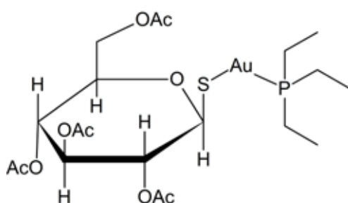
Obr. 1. Štruktúrny vzorec auranofinu
