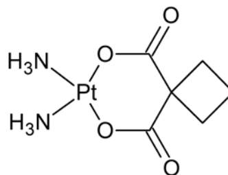
Obr. 5. Štruktúra karboplatiny
