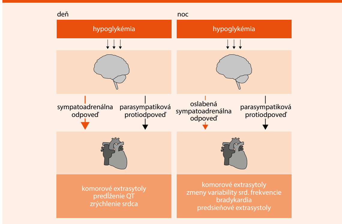
Schéma. Predpokladané mechanizmy hypoglykémiou indukovaných arytmii počas dňa a noci u pacientov s DM2T a s KV chorobami alebo s dvoma KV rizikovými faktormi. Spracované podľa [5]
